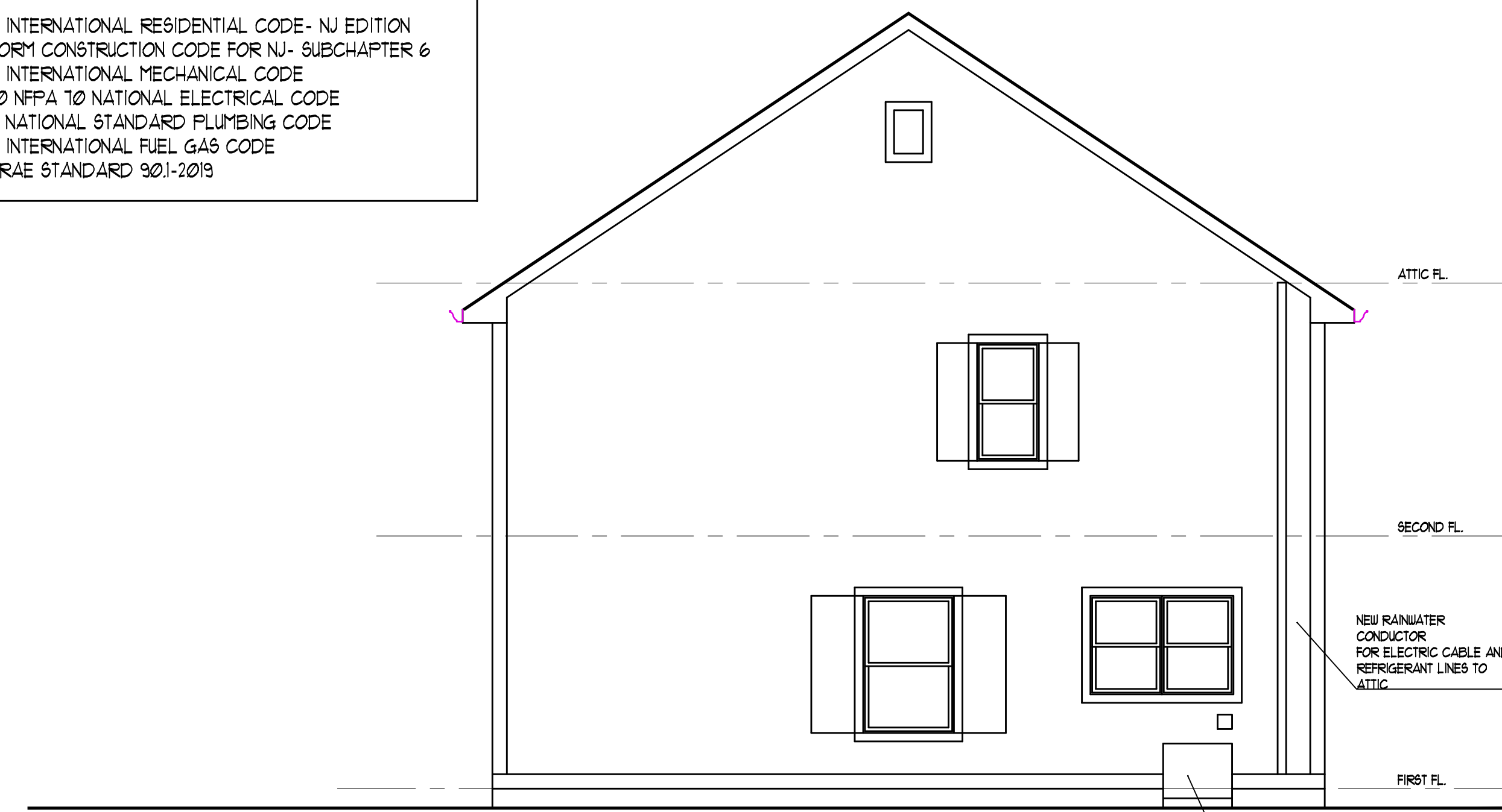
SIDE ELEV. SCALE: 1/4" = 1'-0"
