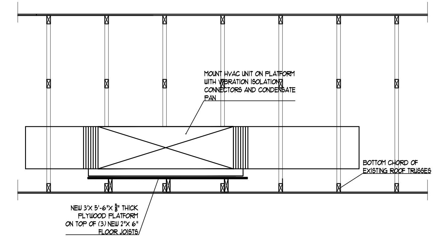
DETAIL 1 SCALE: 1/4" = 1'-0" A3
