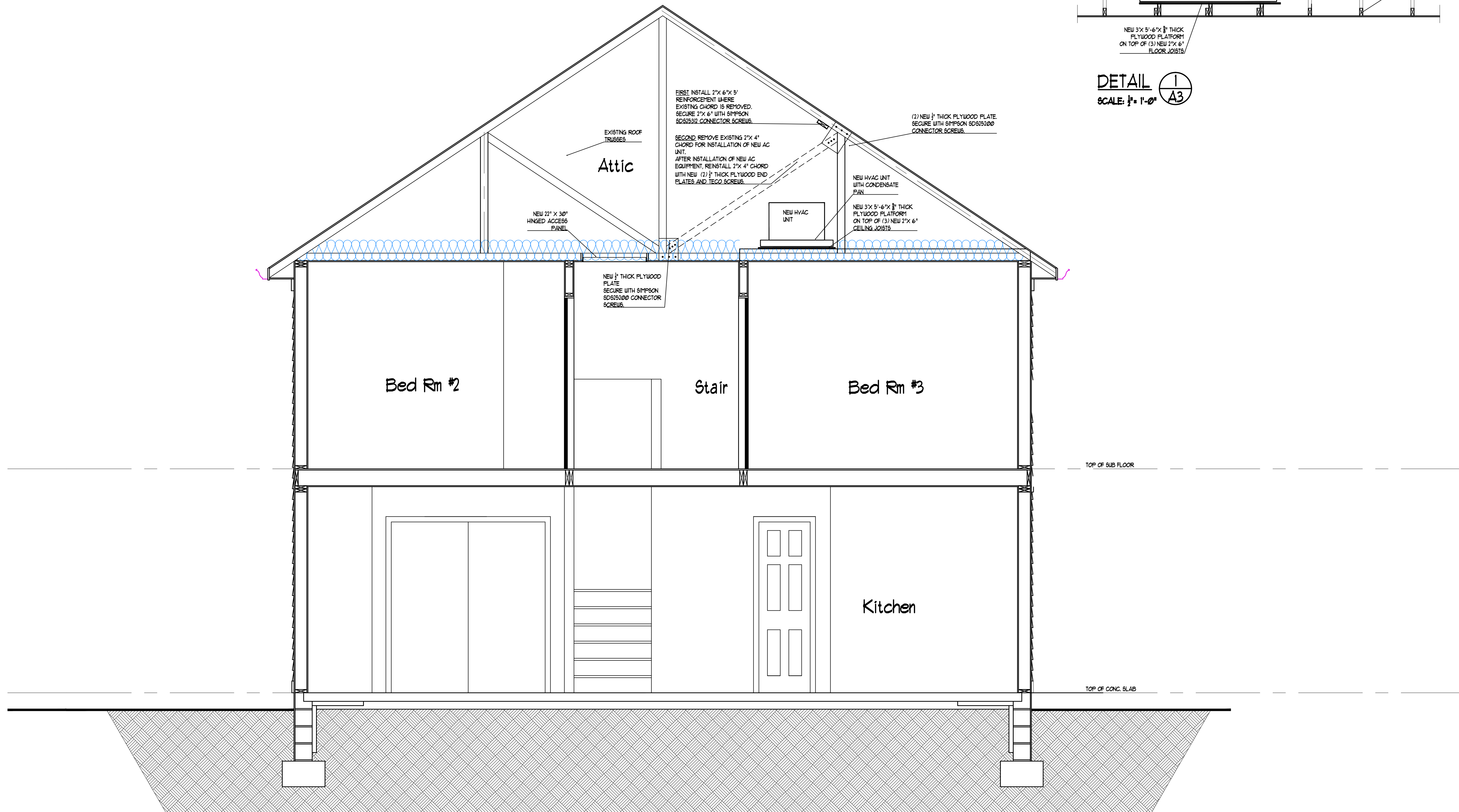
SECTION A-A SCALE: 1/4" = 1'-0"
